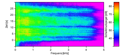
Frequenzverlauf
