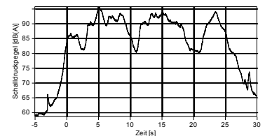
Schallpegelverlauf
